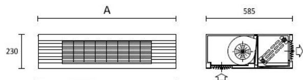
FE-MH
