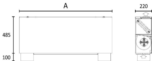
FE-MV
